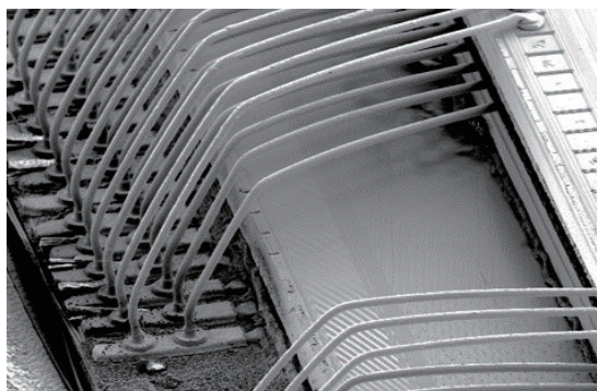
Agワイヤ使用ICパッケージの樹脂開封例
